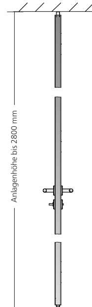
6 Höhenschnitt Front
