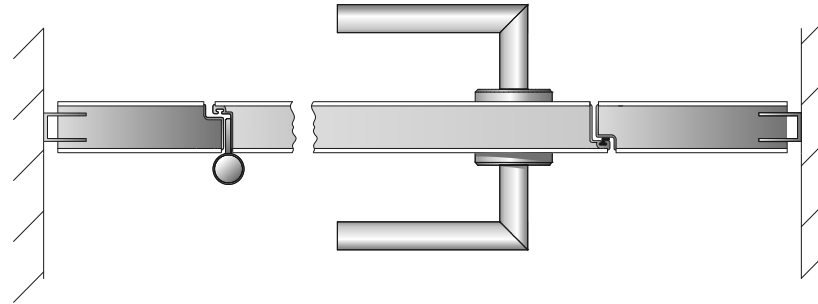
6 Höhenschnitt Front
