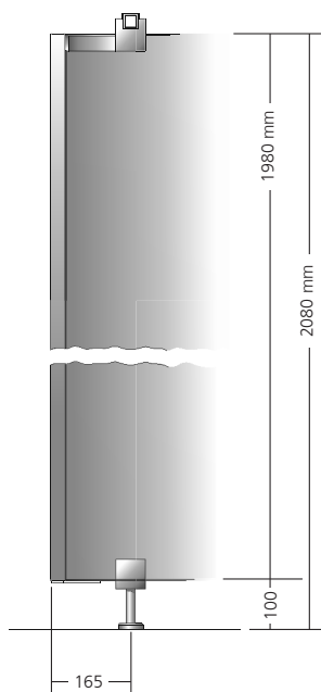
Sezione verticale
