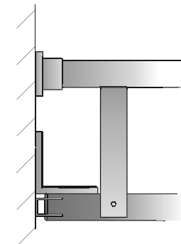
1 Fissaggio profilo superiore a parete
