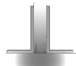
3 Fissaggio interno parete (parete divisoria - parete frontale) con staffe di fissaggio in alluminio all'interno della cabina
